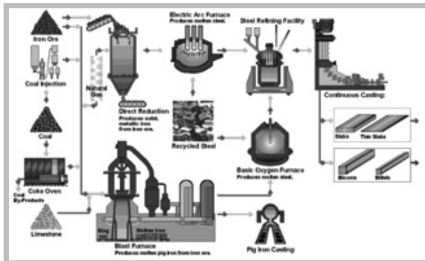
La grafica muestra el proceso de producción de acero, empezando con las materias primas básicas: mineral de hierro y carbón mineral, con sus sub-productos coque y piedra caliza. Se pasa posteriormente al Alto Horno (Blast Furnace), que es el proceso de AHMSA de Monclova o a Reducción Directa, que es el proceso de HYLSA de Monterrey. En el caso de AHMSA, el proceso sigue hacia la producción de arrabio o acero sucio (en inglés pig iron- acero de cochinos) en Horno BOF (Basic Oxygen Furnace), y en el caso de HYLSA el proceso continúa en Horno Eléctrico. Ambos procesos concluyen en el movimiento de grandes ollas que trasladan el acero líquido hacia el proceso de "colada continua" (continuous casting) y de ahí a la producción de acero en lingotes, que posteriormente lleva a la producción final de aceros planos, laminas, estructuras, riel, aceros no planos, varilla, clavo, malla, tubería, etcétera.
